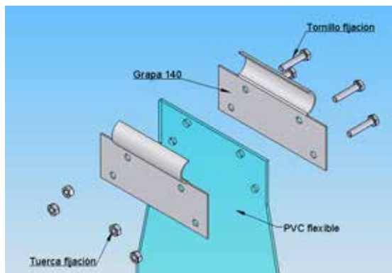
Esquema del sistema de ensamblaje de cortinas PVC
